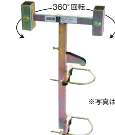
ガードレール支柱用 ●看板適用サイズ:H1400×W280mm ●114φ・140φ ●重量:3.4kg
