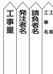
竣工杭(支庁タイプ) ●サイズ:H1800×W90×D90mm 8072202
