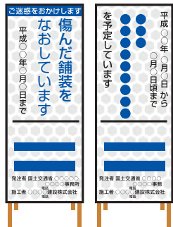
反射材:プリズム高輝度反射シート 色:ホワイト サイズ:(板面)H1400×W550mm
