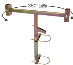
ガードレール支柱用 ●看板適用サイズ:H1400×W550mm ●114φ・140φ ●重量:3.2kg
